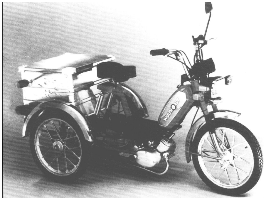
Wulfhorst-Lastendreirad 1987
