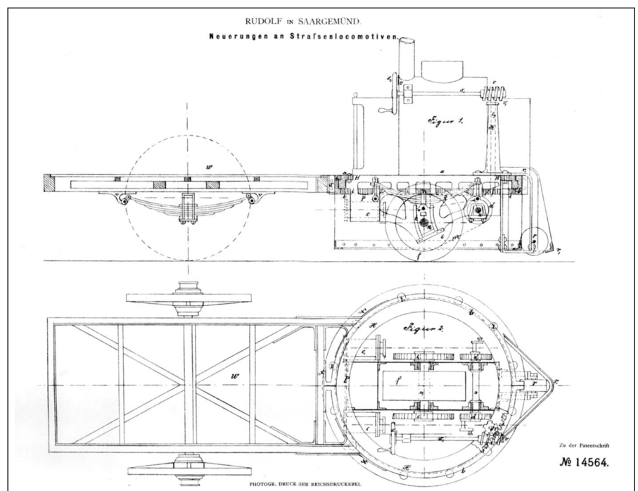
Die Konstruktion der Straßenlokomotive von Herrn Rudolf aus Saargemünd 1880 1
