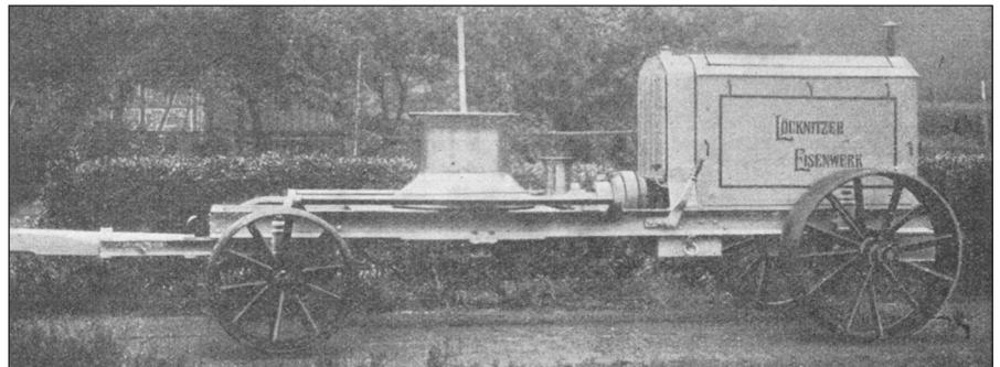
Ankerwagen der Löcknitzer Eisenwerke
