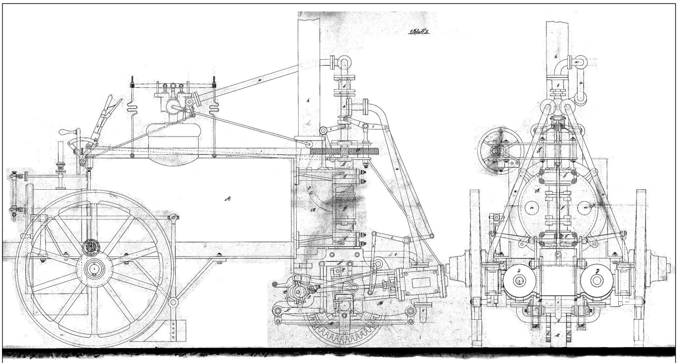
Zeichnung aus dem Antrag vom 20. November 1867 auf ein Patent des Preußischen Königreiches
