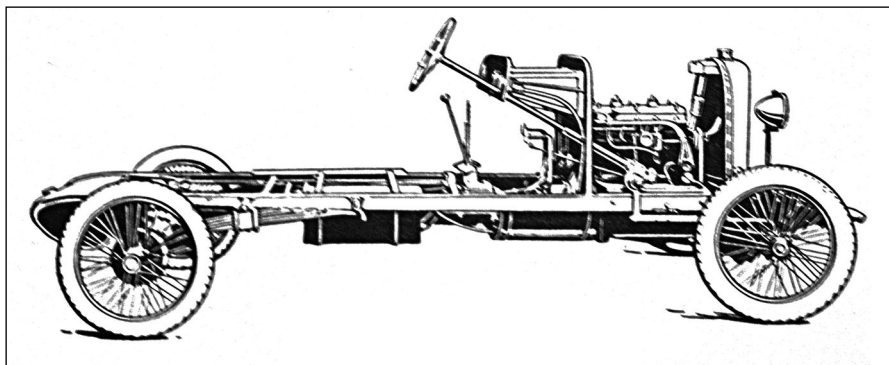
Das rechtsgelenkte 6/30-PS-Alan-Chassis war speziell für Lieferwagen konzipiert 1
